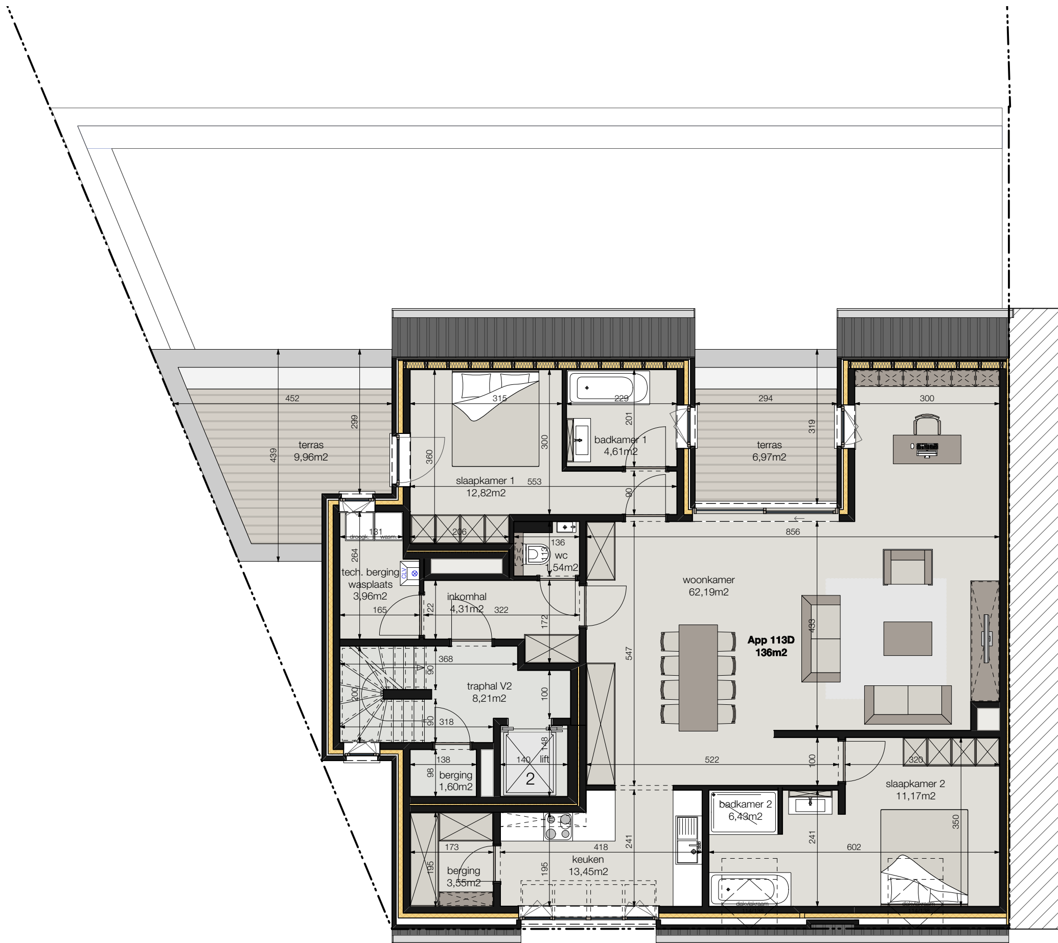
Merelbekestraat Melle -2° verdieping App. 113D
