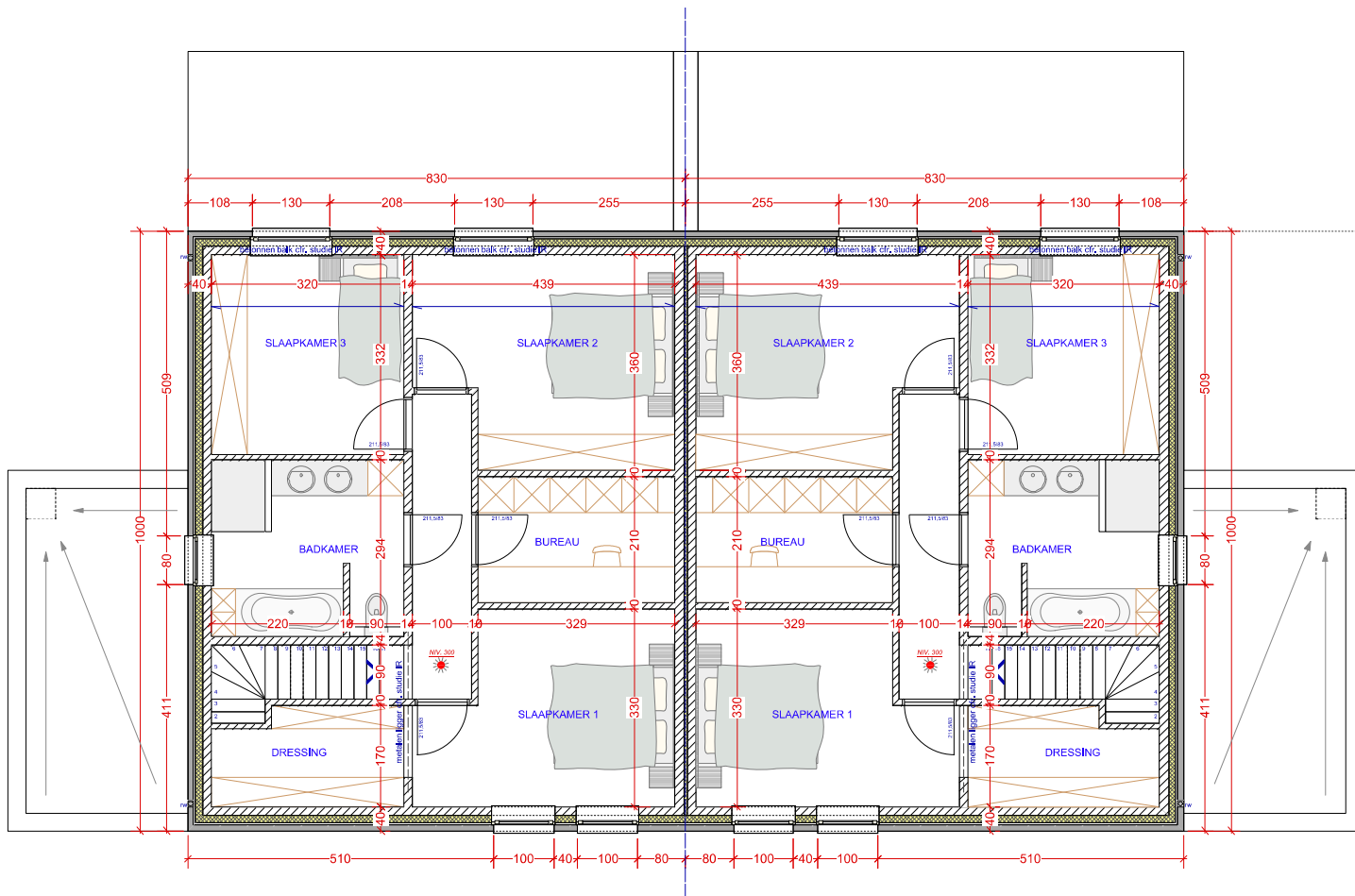
VERDIEPINGSPLAN
